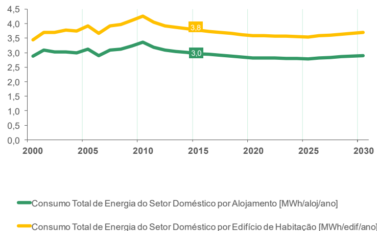
Figura 34 - Consumo Total de Energia do Setor Doméstico por Edifício de Habitação e por Alojamento[MWh/alof/ano] [MWh/edif/ano]
