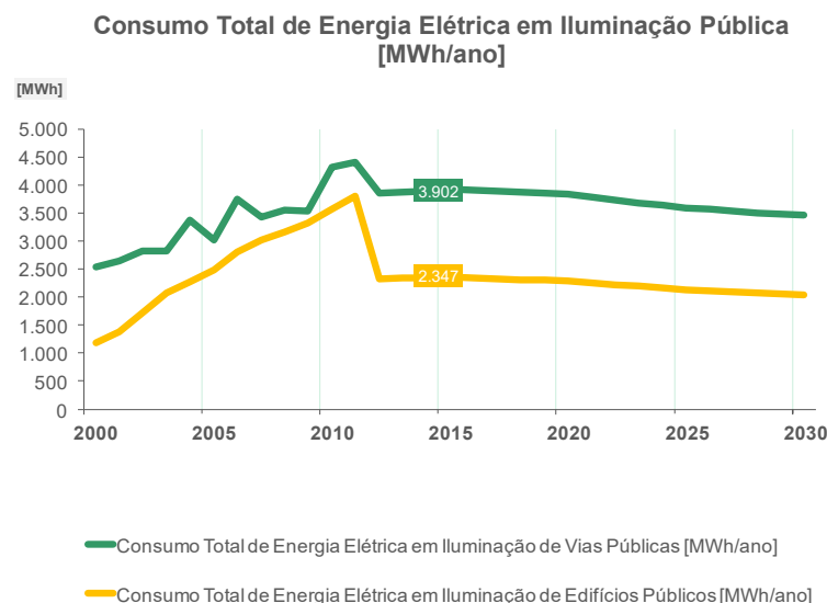
Figura 35 - Consumo Total de Energia Elétrica em Iluminação Pública [MWh/ano]
