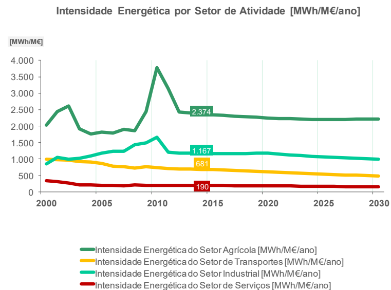
Figura 9 - Intensidade Energética por Setor de Atividade [MWh/M€/ano]
