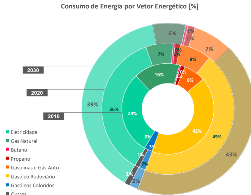
Figura 3 - Consumo de Energia por Vetor Energético em 2010, 2020 e 2030 [%]
