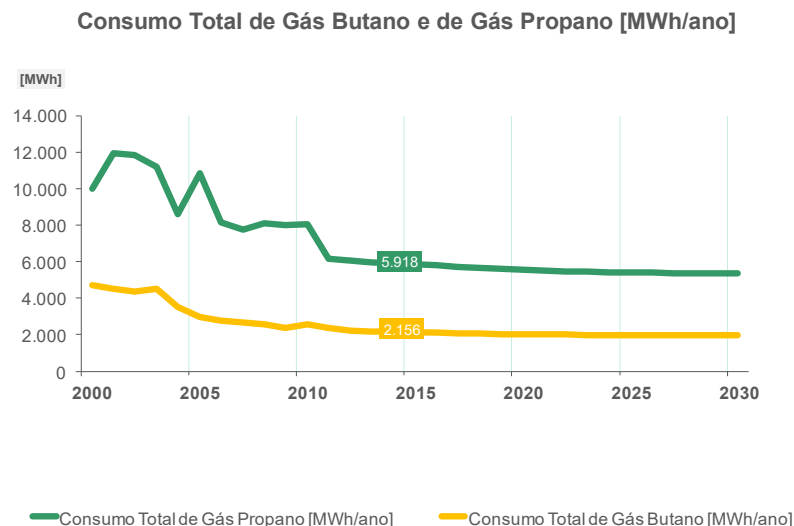
Figura 26 – Consumo Total de Gás Butano e de Gás Propano [MWh/ano]
