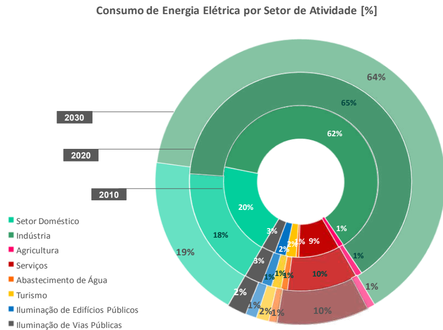
Figura 4 - Consumo de Energia Elétrica por Setor de Atividade em 2010, 2020 e 2030 [%]
